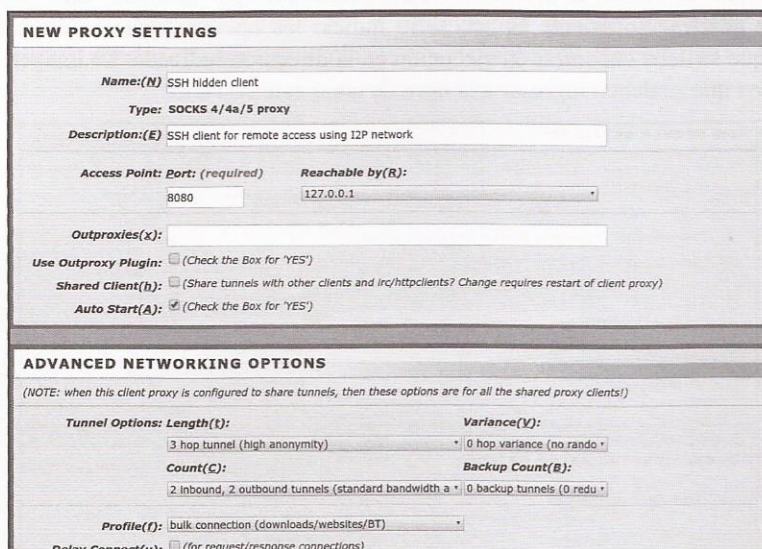
Imagen 02.22: Creación de un túnel cliente SOCKS en I2PTunnel.
